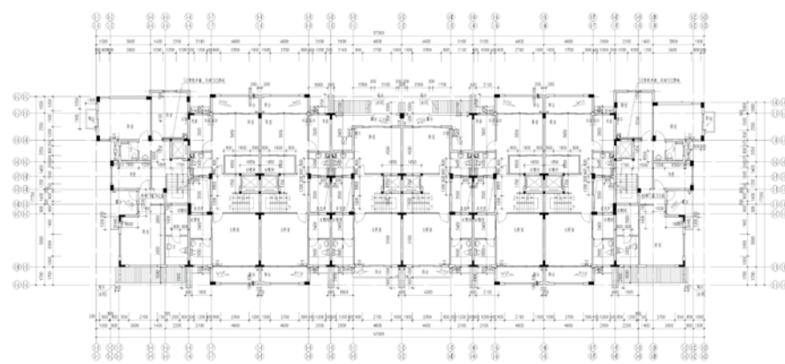
三层平面图 Third Floor Plan
